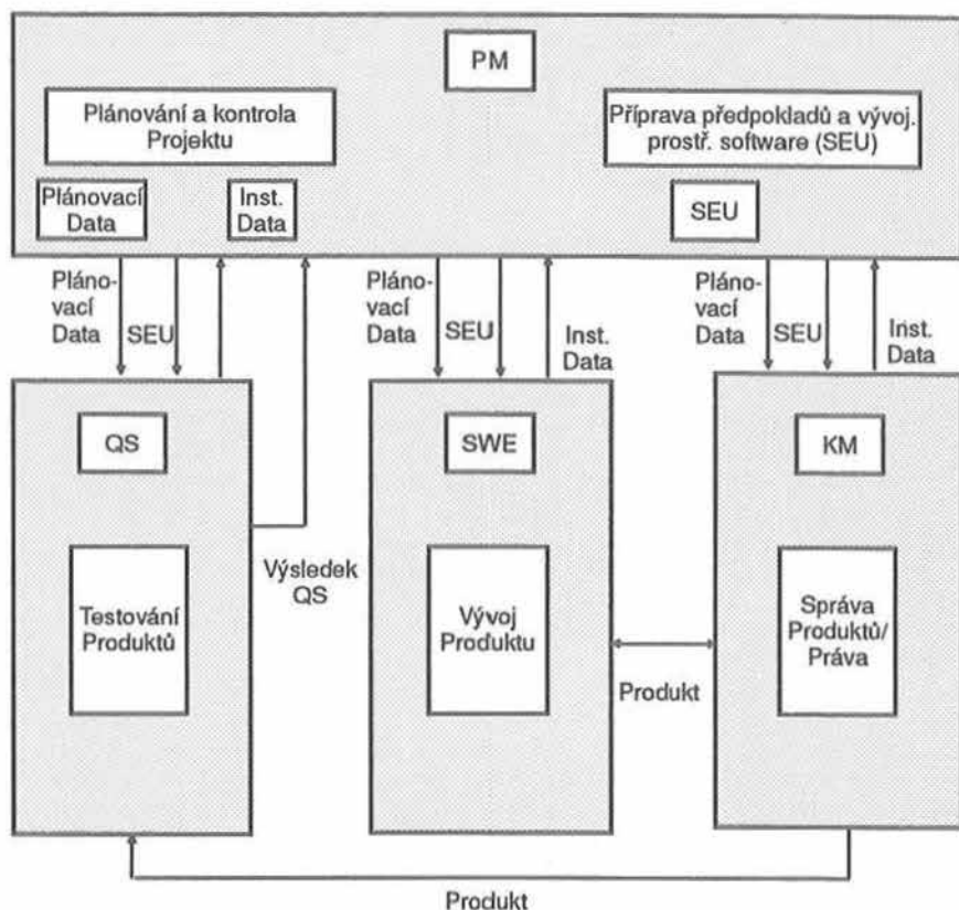
Obr. 2 Činnosti provádějící vypracování software
