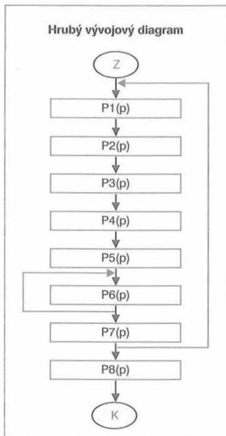
Obr. 1: Procedury klouzavého řízení OVV ve vývojovém diagramu
