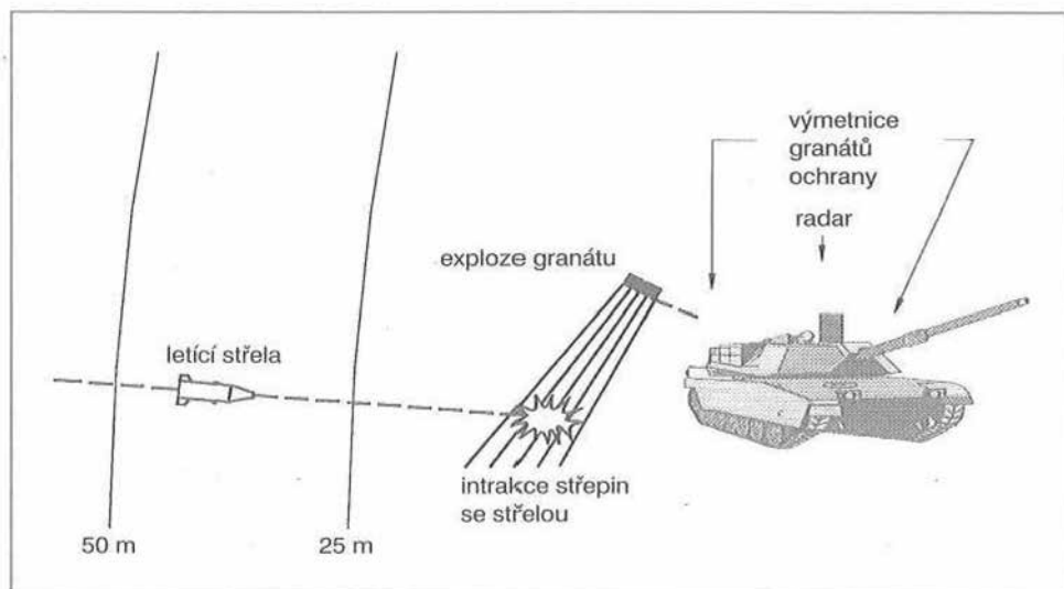
Obr. 2: Schéma činnosti systému APS ARENA
