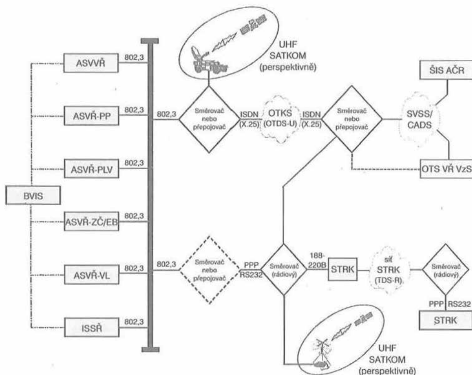
Obr. 9: Konfigurace vyjadřující síťový přístup v OTS
