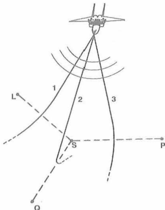
Symbolické znázornění možné konfigurace PSS a principu 3D měření souřadnic polohy cíle metodou protínání tří hyperbol.
