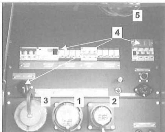
Obr. 6: Osazení schrány vstupních zdrojů
