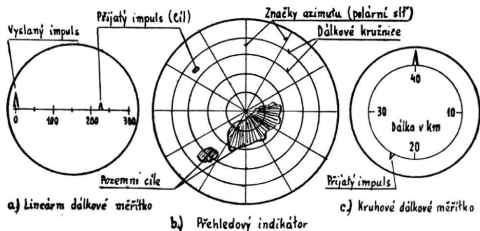
Obr. 6. Stínítka obrazových elektronek
