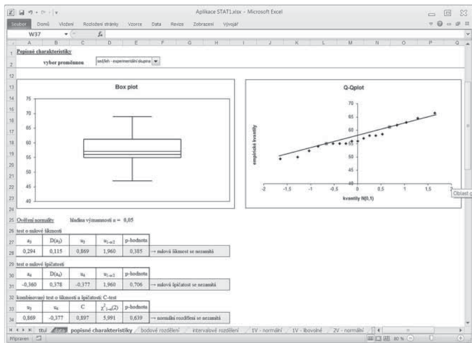
Obr. 3: Ověření normality
