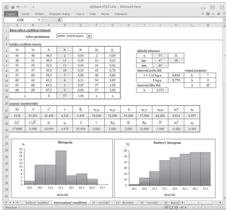
Obr. 2: Intervalové rozdělení četností a výběrové charakteristiky
